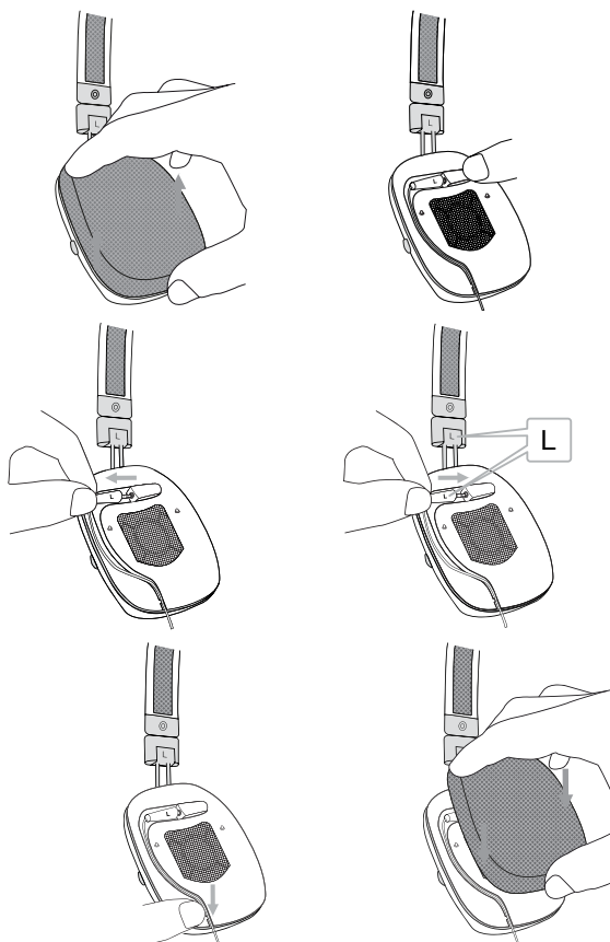
Obrázek 4 Výměna kabelu
