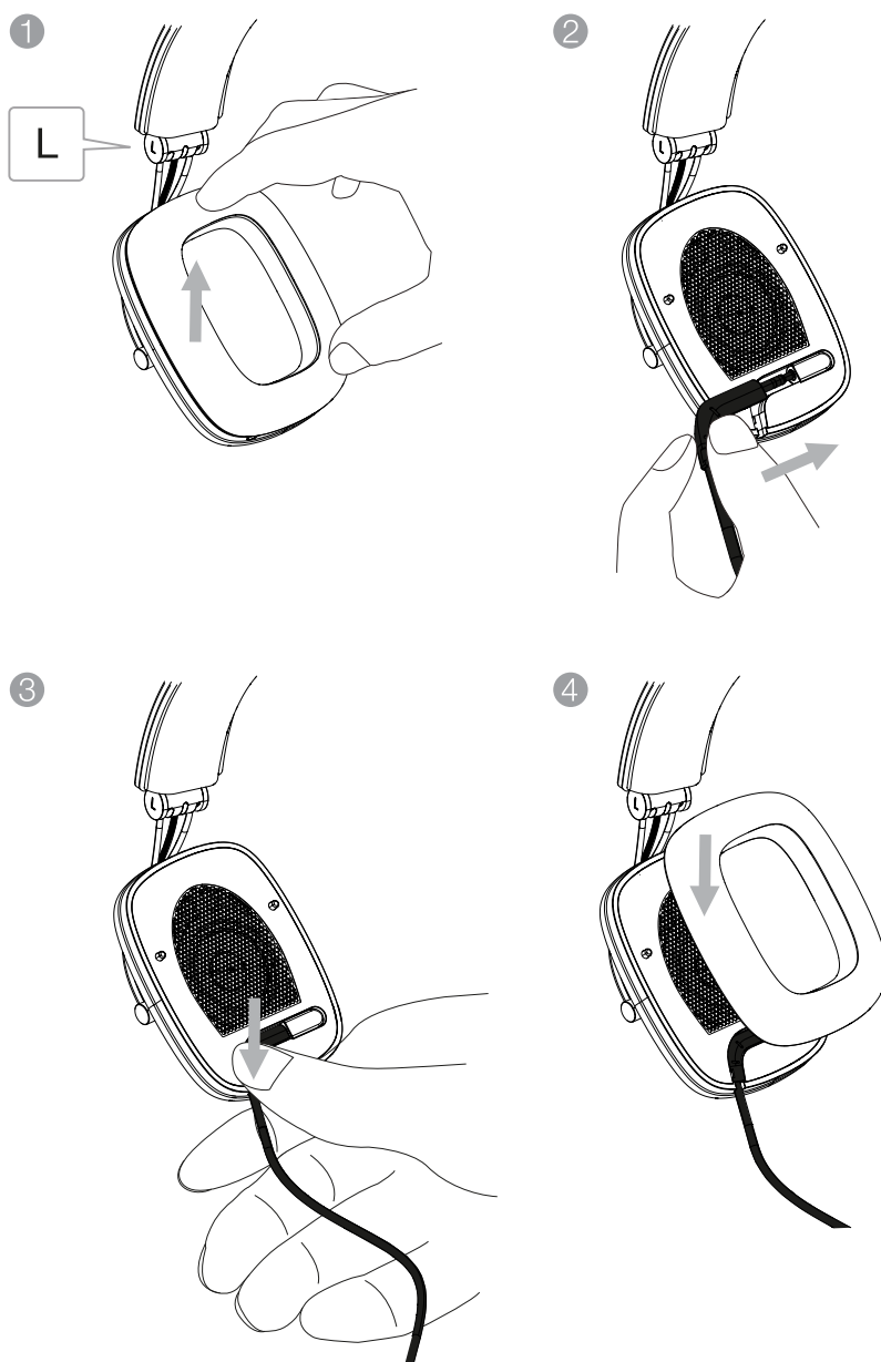
Diagrama 5 Colocación del cable de audio
